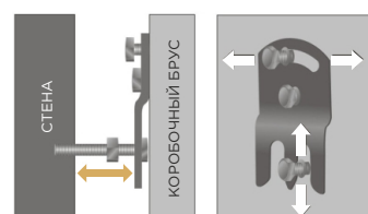
Монтажный комплект для установки дверей СК-1
